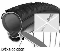
Rys. 4/44 Źródło Schwalbe
