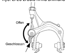
Dźwignia szybkozamykacza
