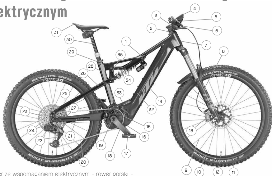
Rower ze wspomaganiem elektrycznym – rower górski – pełne zawieszenie (przykładowy nadruk symbolu)
