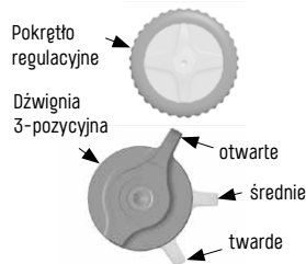
Rys. 1/48 Tłumienie przy ugięciu amortyzatora źródło: Fox
