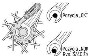
Rys. 3/40 Źródło firma Shimano
