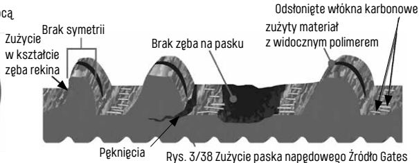
Rys. 3/38 Zużycie paska napędowego Źródło Gates
