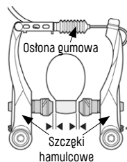
Rys. 3/28 Źródło firma Shimano
