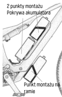
Rys. 1/ Przykłady punktów montażu w rowerze ze wspomaganiem elektrycznym
